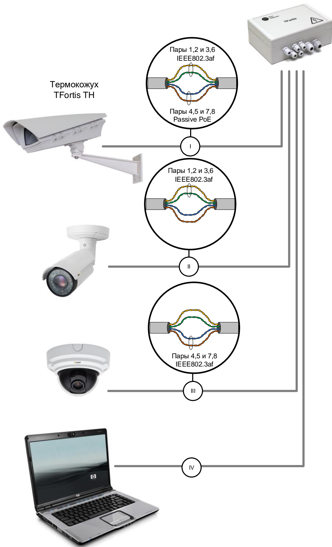
Рисунок 2.3. Схема питания по PoE для разных случаев
