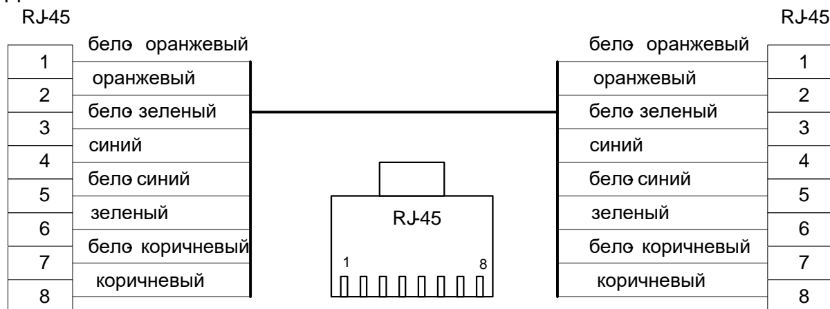
Рисунок 6.4 - Разделка кабеля.
