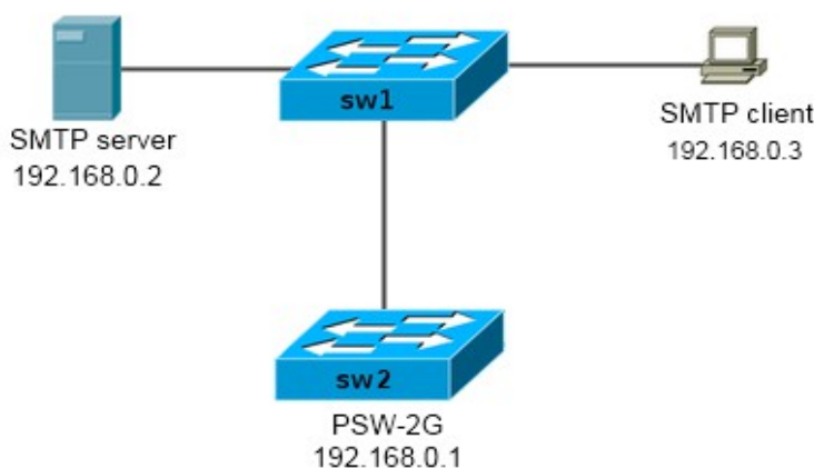
Рис. 5.3.12.1.1 Структура сети
