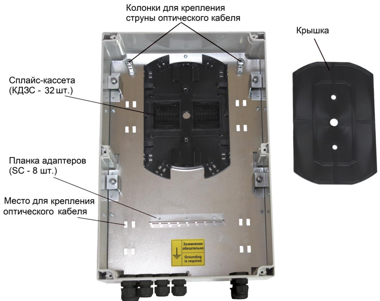
Рисунок 3.4 - Оптический кросс
