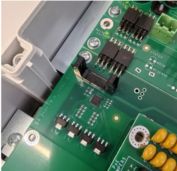
Рисунок 3.5.1 - Датчика вскрытия на плате
