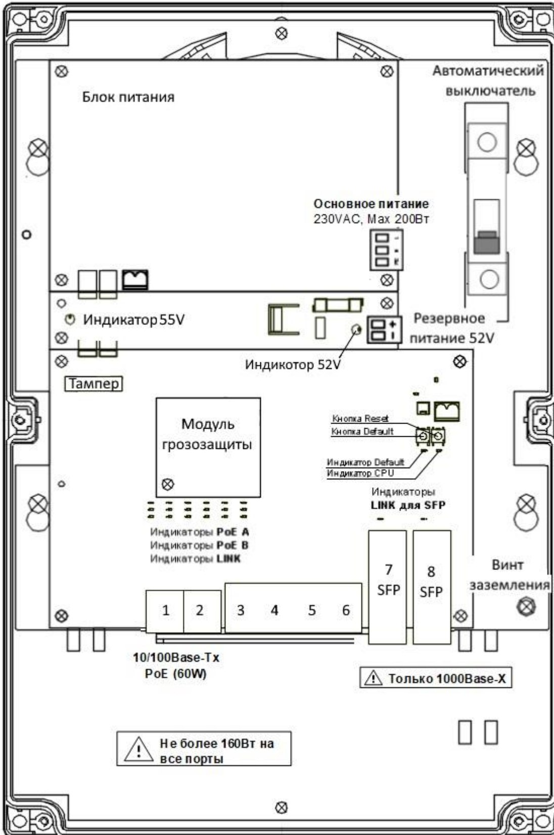
Рисунок 3.2 - Расположение элементов коммутатора PSW -2G6F+
