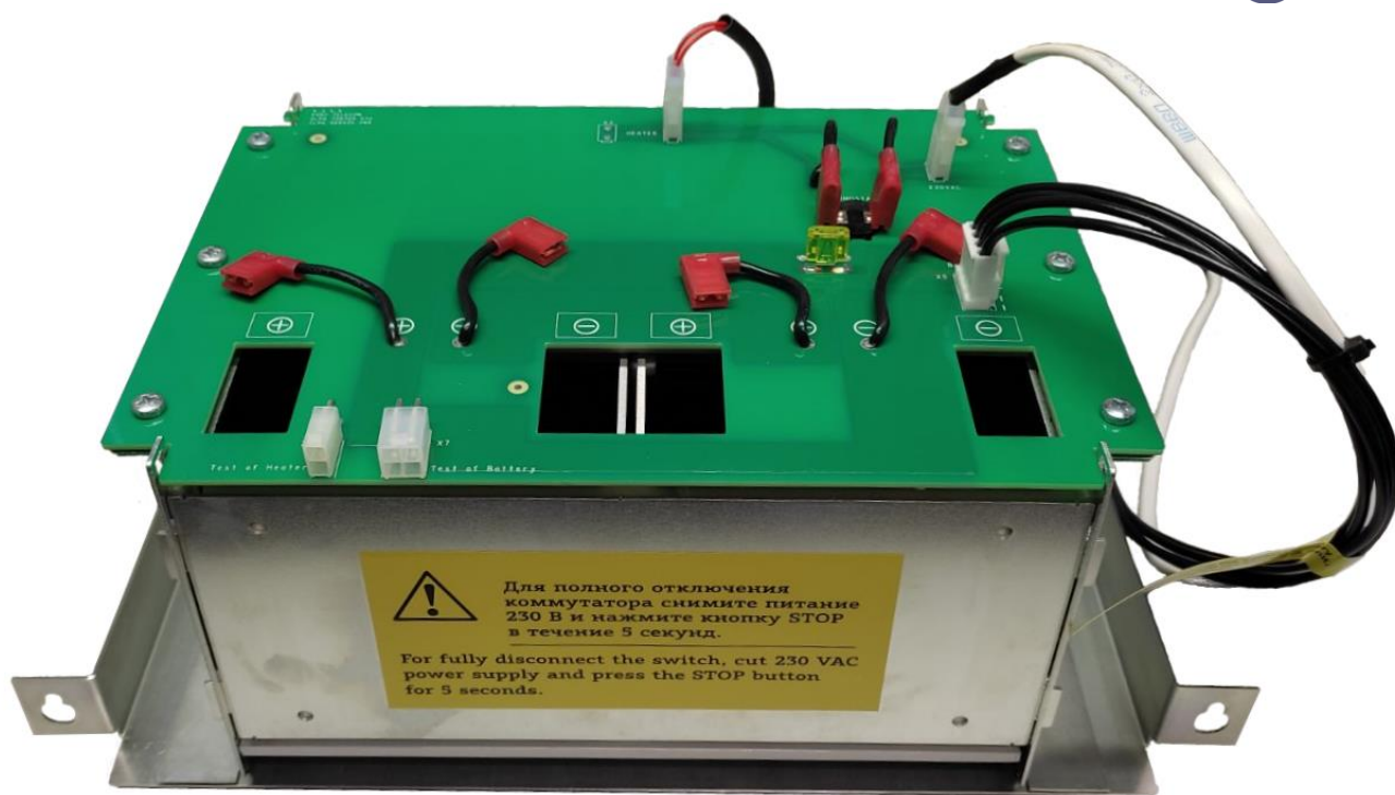
Рисунок 3.6 – отсек АКБ.
