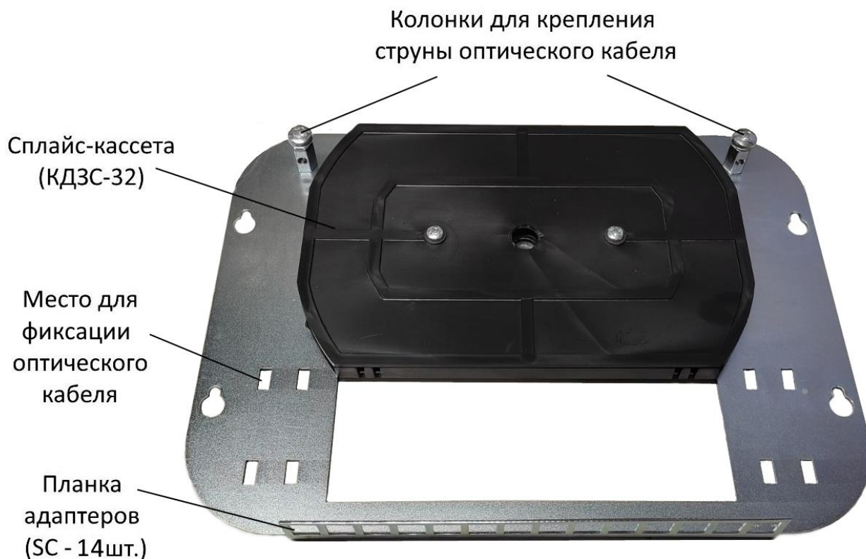
Рисунок 3.3 - Оптический кросс.
