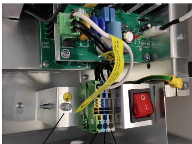
Винт заземления PE N L
