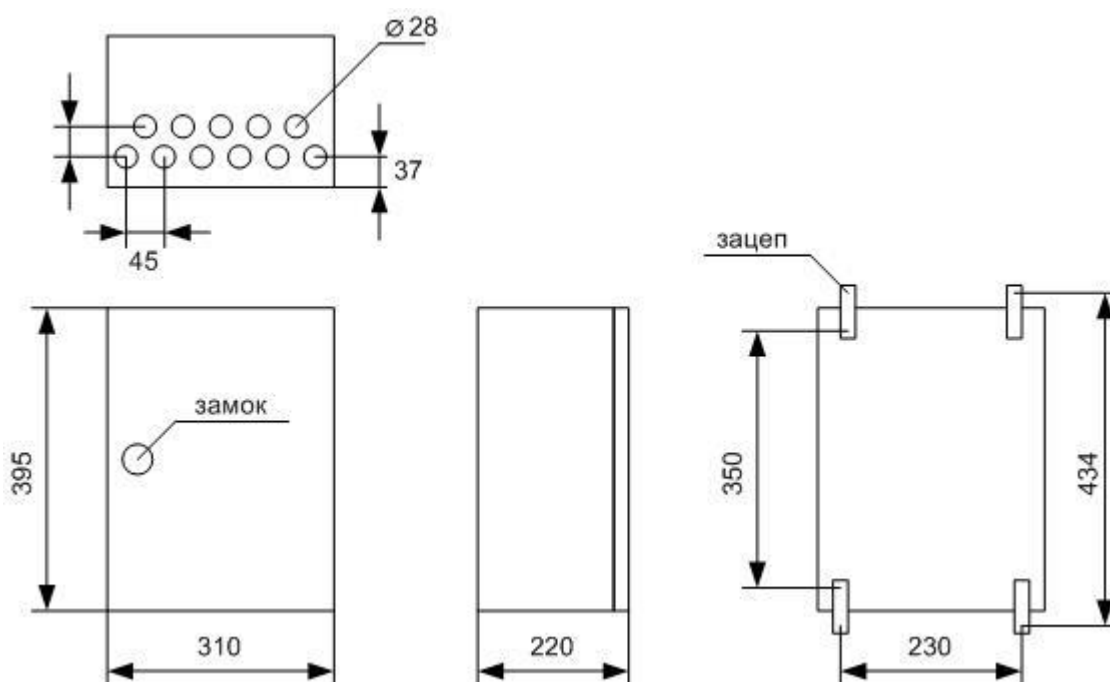
Рис. 8. Чертеж
