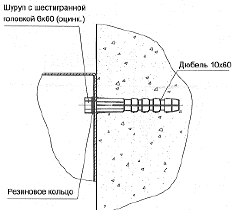
Рис. 6. Установка на стену без зацепов
