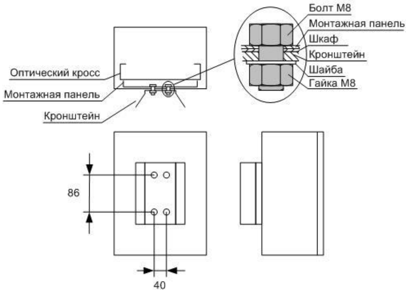
Рис. 5. Установка кронштейна для крепления шкафа на опору
