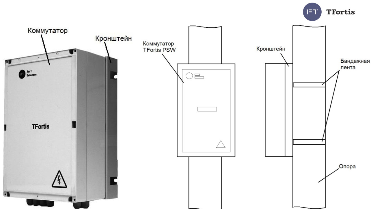
Рисунок 7.2 - Монтаж коммутатора на Кронштейн для PSW.
