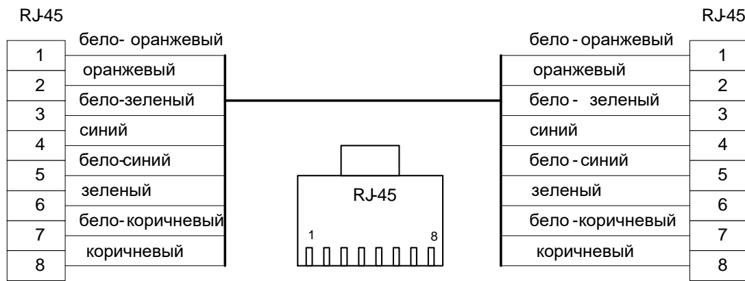
Рисунок 7.4 - Разделка кабеля.
