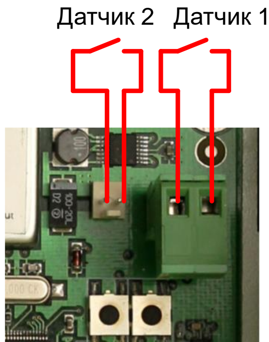
Рисунок 3.6 - Сухие контакты
