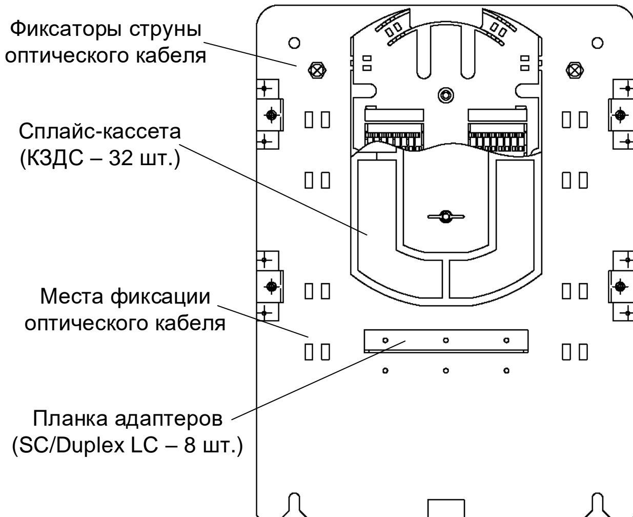
Рисунок 3.4 - Оптический кросс
